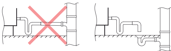
Abb. 12b. Anschluss des Kondensatablaufs an die Kanalisation
