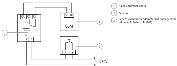
Abb. 16. Beispiel für die Aktivierung des Lüftungsmodus „Übersteuerung“ bei Verwendung einer zusätzlichen Absaugung mit einer motorisierten Klappe (siehe Abb. 10)
