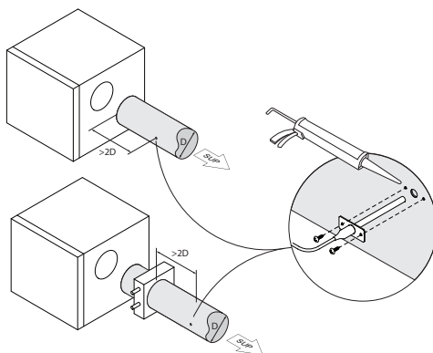
Abb. 15b. Installation eines Zulufttemperaturfühlers
