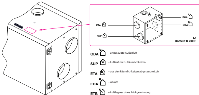
Abb. 9. Kennzeichnung der Luftkanäle
