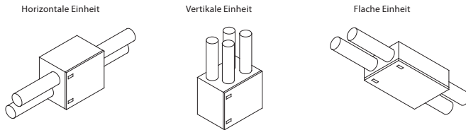
Abb. 1. Klassifikation der Einheiten nach Kanalanschluss
