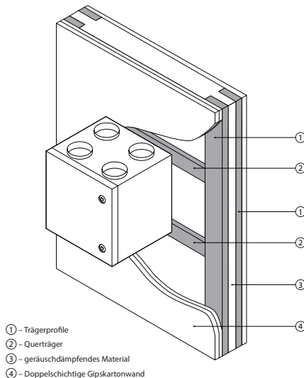
Abb. 8. Anbringung der Einheit an einer Gipskarton-Trennwand
