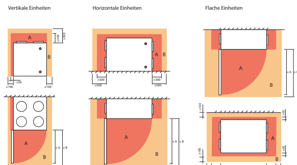
Abb. 5. Minimaler Raum für Wartung
