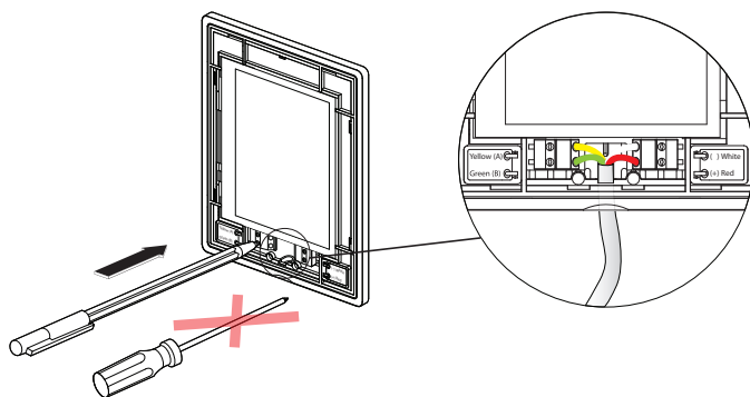
Abb. 18. Kabelverbindung zum Bedienfeld
