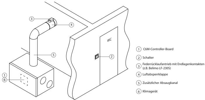
Abb. 10. Beispiel für die Montage eines zusätzlichen Abluftkanals
