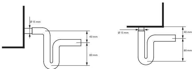
Abb. 12a. Installation eines Siphons ohne Einwegventil
