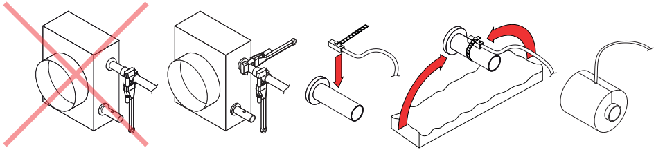
Abb. 11. Anschließen der Wassererhitzer-/Kühlerschläuche und Installation des Wassertemperaturfühlers
