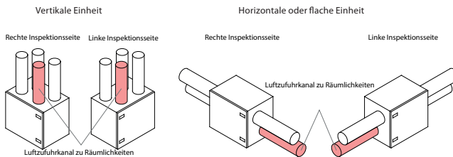
Abb. 2. Klassifikation der Einheiten nach Inspektionsseite
