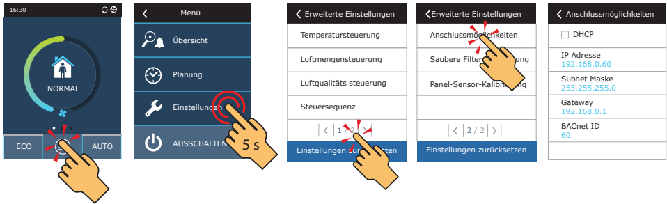
Abb. 19. Anzeigen und Ändern der IP-Adresse des RLT-Geräts auf dem Bedienfeld
