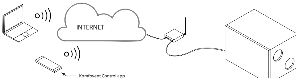
Abb. 21. Beispiele für den Anschluss des Geräts an ein lokales Netzwerk oder das Internet
