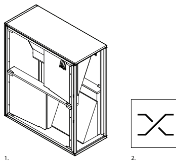
Abb. 12. Luftaustauschabschnitt
