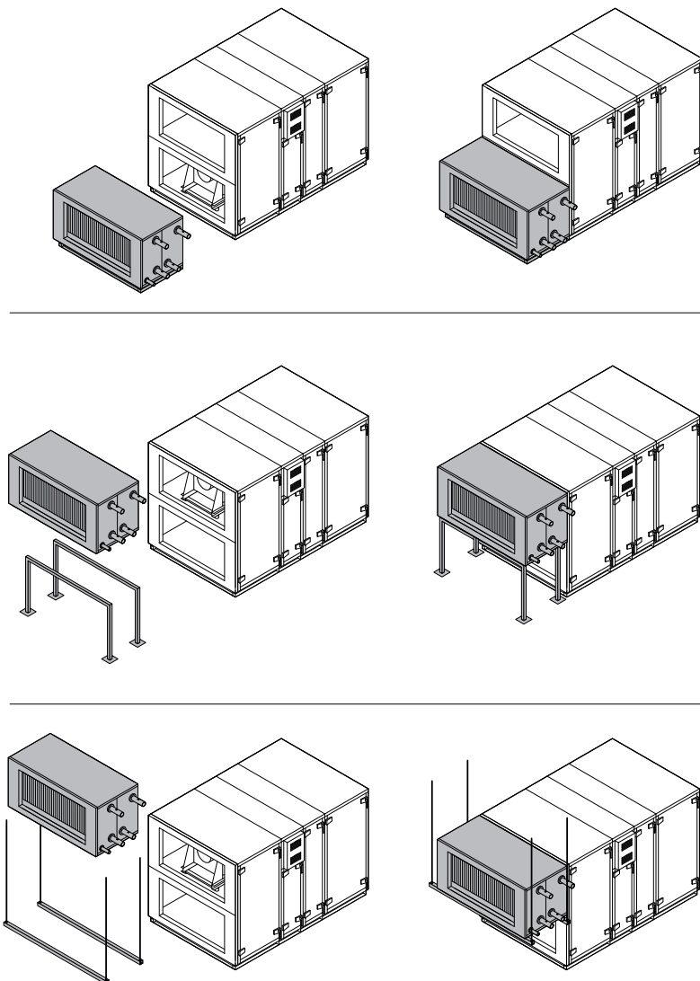
Abb. 25. Beispiele für die Installation von Heiz-/Kühlabschnitten
