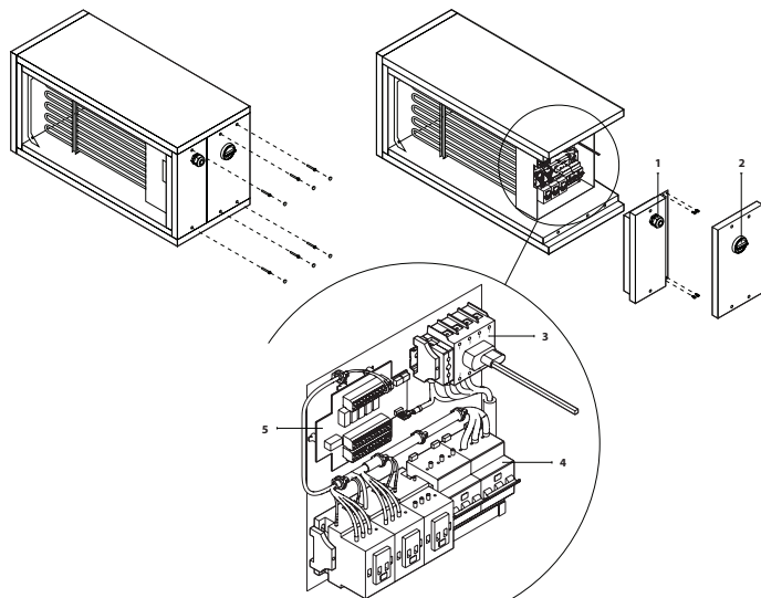
Abb. 37. Haupttrennschalter in elektrischem Heizabschnitt 1 – Zuleitungskabeldurchführung, 2 – Griff des Haupttrennschalters, 3 – Haupttrennschalter, 4 – Sicherung, 5 – elektronische Heizungssteuertafel
