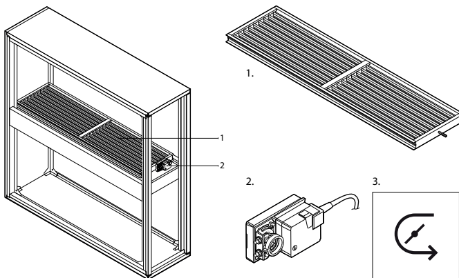
Abb. 5. Abschnitt Umluftsteuerung
