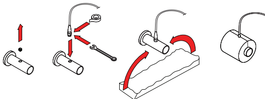
Abb. 28. Installation eines Rücklaufwassertemperaturfühlers mit Gewinde 3
