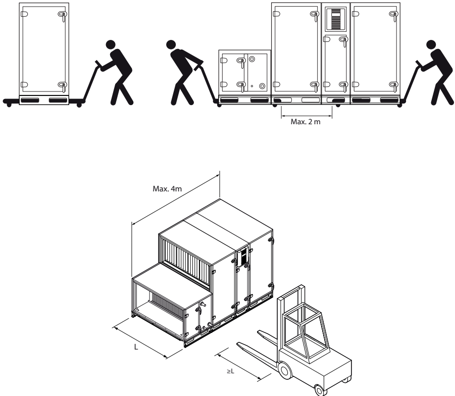
Abb. 13. Transport der Anlage mit einem Gabelstapler oder einem Rollwagen
