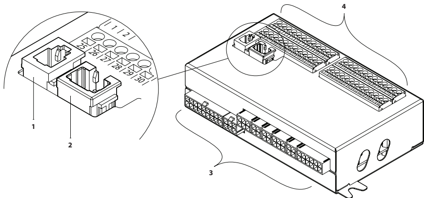
Abb. 39. Hauptplatine des C5-Bedienfeldes
