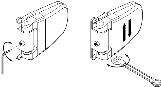
Abb. 21. Einstellen der Scharniere
