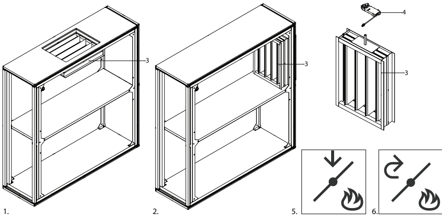
Abb. 11. Abschnitt Rauchabzug
