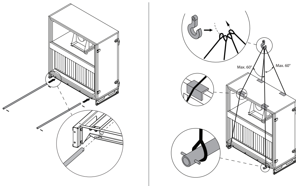
Abb. 14. Anheben einzelner Abschnitte 1
