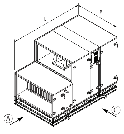
Abb. 16. Im Werk vormontierte Gerätemontagerahmen
