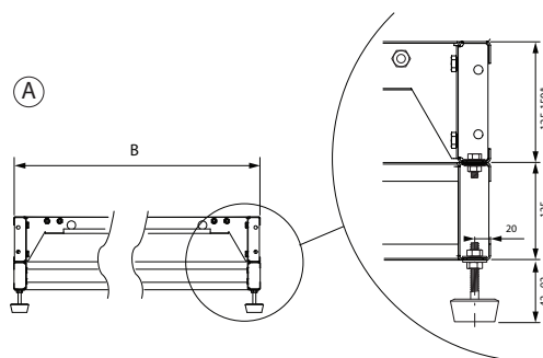
Abb. 17. Abmessungen des verstärkten Montagerahmens
