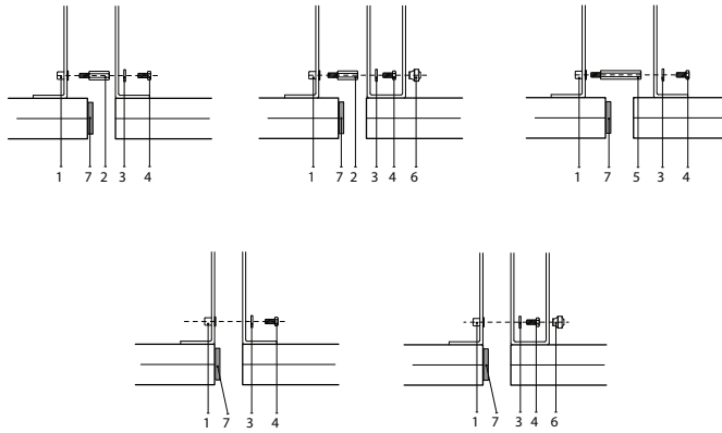
Abb. 23. Arten von internen Abschnittsverbindungen 1 – Gewindebuchse, 2 – Distanzstück 35 mm, 3 – Unterlegscheibe, 4 – Schraube M6, 5 – Abstandhalter 70 mm, 6 – Tülle d29, 7 – Klebe-Dichtung
