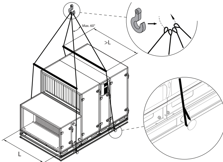
Abb. 15. Vollständig montierte Lüftungsanlage auf verstärkten Sockelrahmen heben 1
