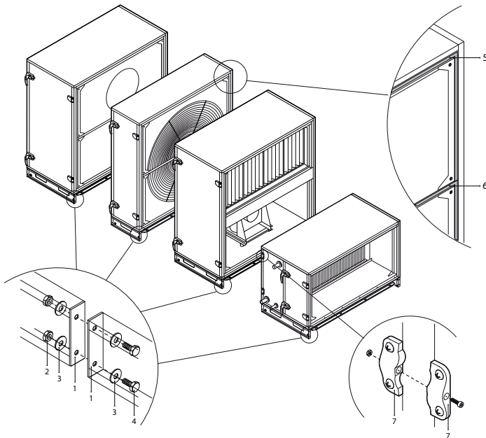
Abb. 22. Äußerer Anschluss und Abdichtung der Abschnitte
