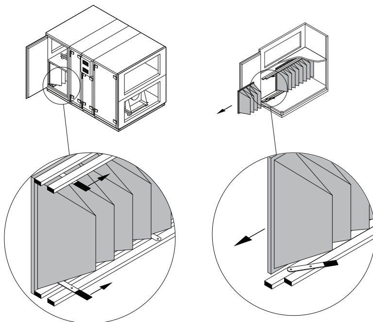
Abb. 56. Filter-Klemmvorrichtung
