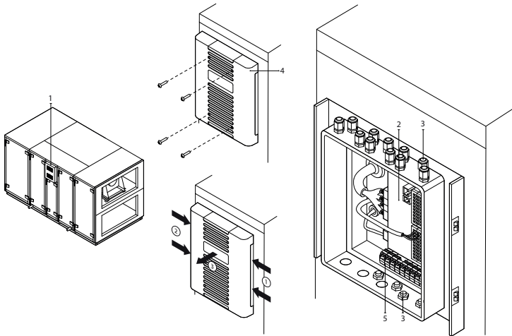
Abb. 38. Steuerungsbox
