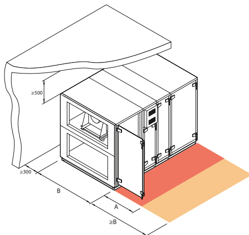
Abb. 19. Inspektionsbereich für Geräte
