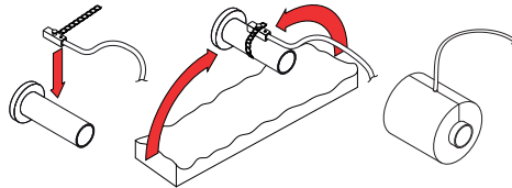
Abb. 27. Installation eines oberflächenmontierten Rücklauf-Wassertemperaturfühlers 2
