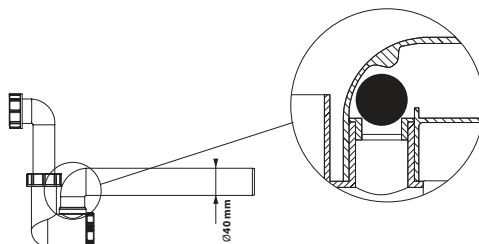
Abb. 30. Beispiel eines Siphons mit Rückschlagventil
