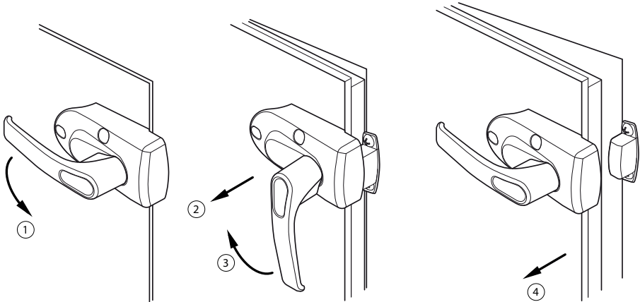
Abb. 20. Öffnen der Tür
