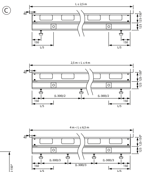
Abb. 16. Im Werk vormontierte Gerätemontagerahmen
