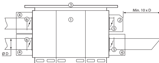
Abb. 34. Zubehör für außen installierte Geräte
