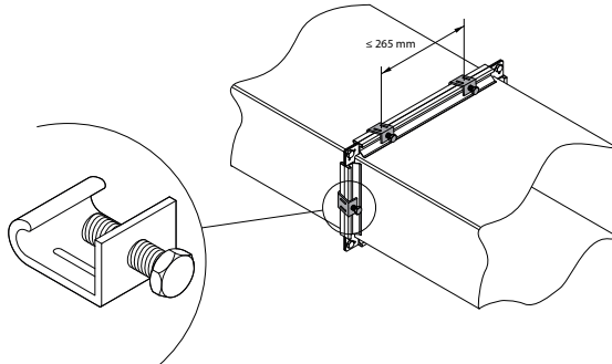
Abb. 33. Beispiel für eine Kanalverbindung mit Kanalklammern
