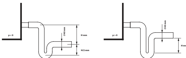
Abb. 29. Installation eines Siphons ohne Rückschlagventil
