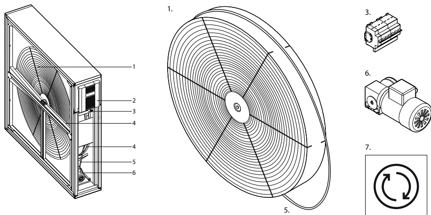
Abb. 3. Abschnitt Rotierender Rekuperator
