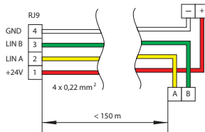
Abb. 49. Anschlussplan für das Bedienpanel
