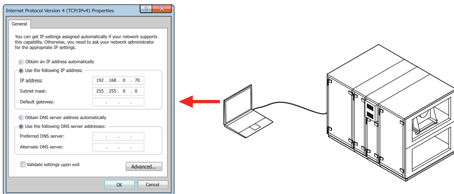
Abb. 54. Computernetzwerkeinstellungen für den direkten Anschluss an das Gerät
