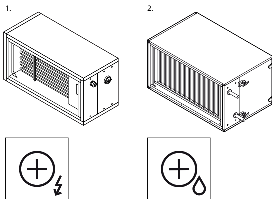
Abb. 7. Abschnitt Erhitzer
