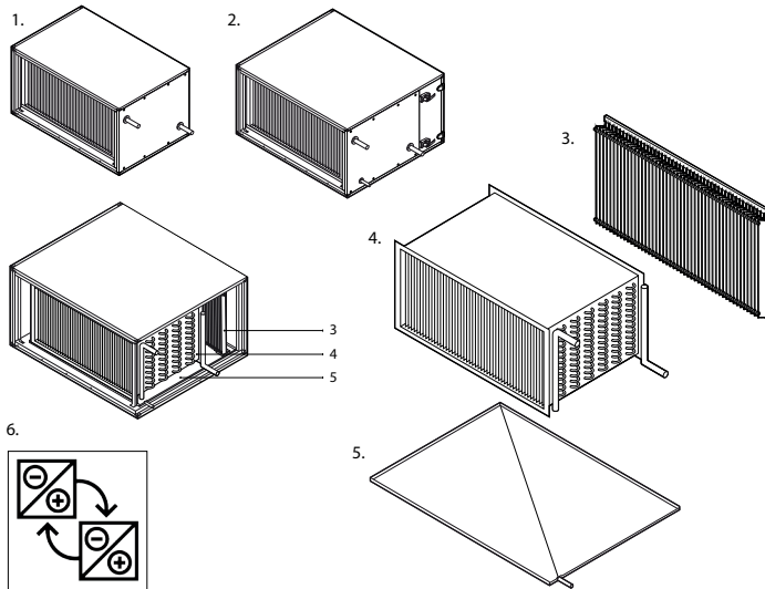
Abb. 4. Auswahl flüssigkeitsgekoppelter Wärmetauscher
