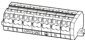
Abb. 45. Zusätzlicher Anschlussklemmenblock
