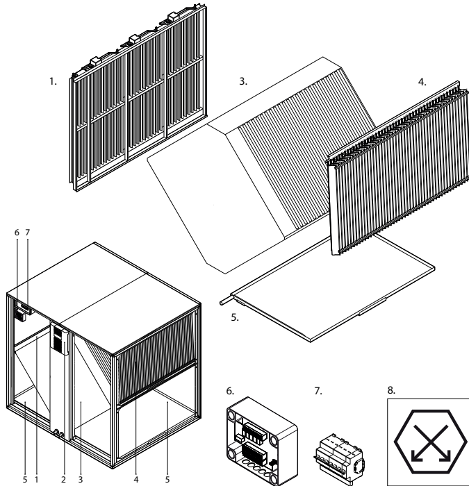
Abb. 2. Gegenstrom-Wärmetauscher (CF)-Abschnitt
