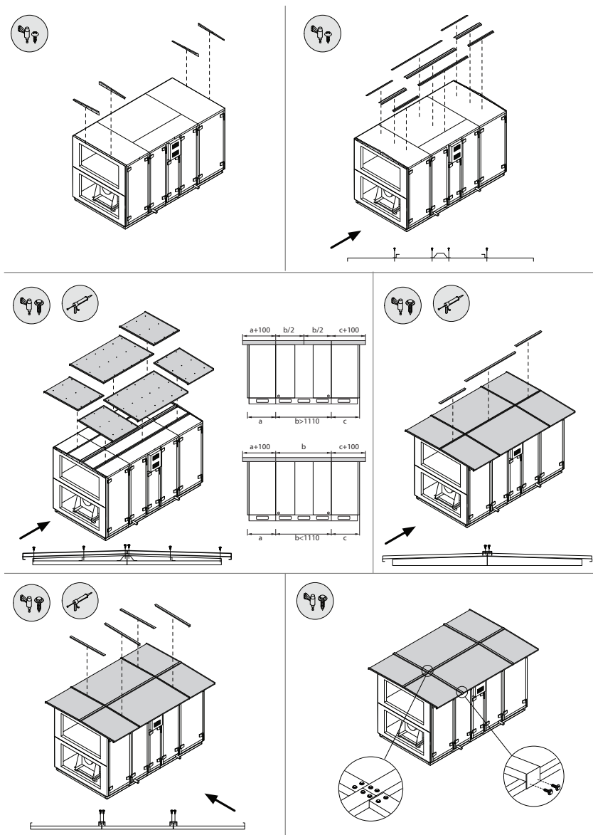
Abb. 35. Installation eines zusätzlich bestellten Schutzdachs 1
