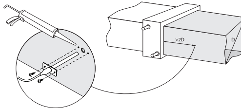
Abb. 44. Installation eines Zulufttemperaturfühlers
