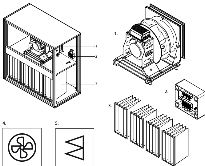
Abb. 1. Filter-Ventilator-Teil
