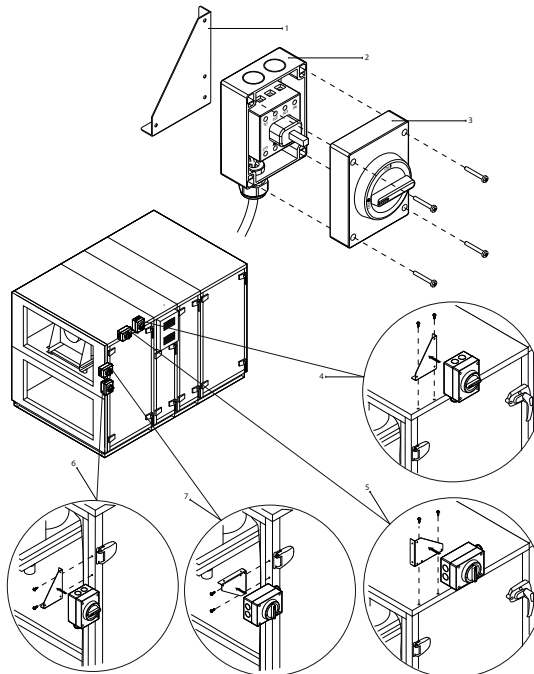
Abb. 36. Hauptleistungsschalter und Montagebeispiele
