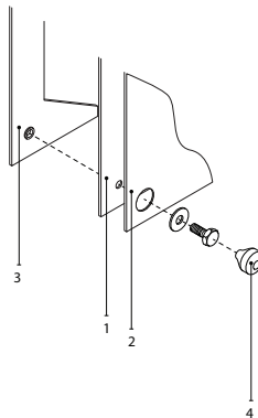
Abb. 24. Interne Verbindung in einem Ventilatorabschnitt 1 – Winkelstück zur Befestigung des Lüfterteils, 2 – Wand, an der der Lüfter montiert ist, 3 – Spannwinkel für anderen Abschnitt, 4 – Tülle d29
