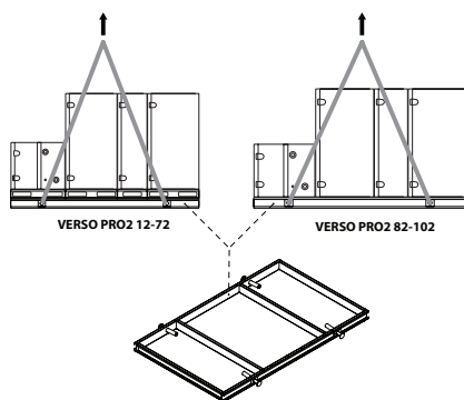
Abb. 16. Im Werk vormontierte Gerätemontagerahmen
