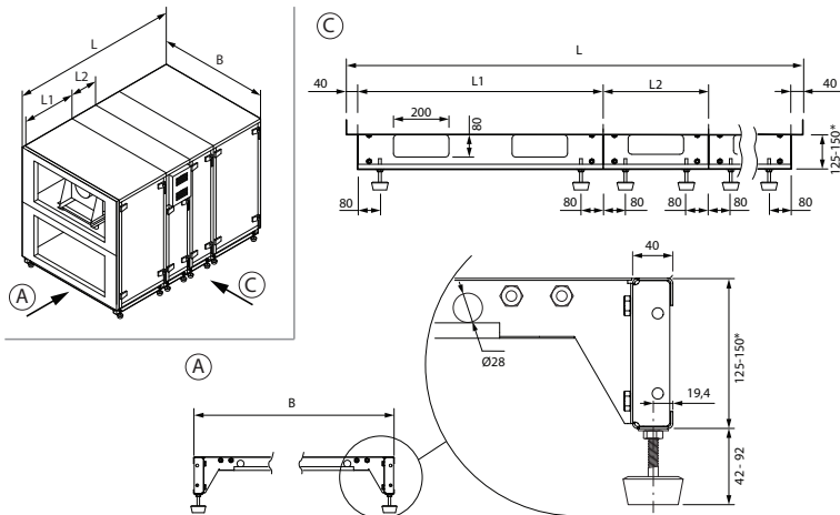
Abb. 18. Einbaurahmen mit verstellbaren Füßen
