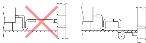
Abb. 31. Anschluss des Kondensatablaufs an die Kanalisation
