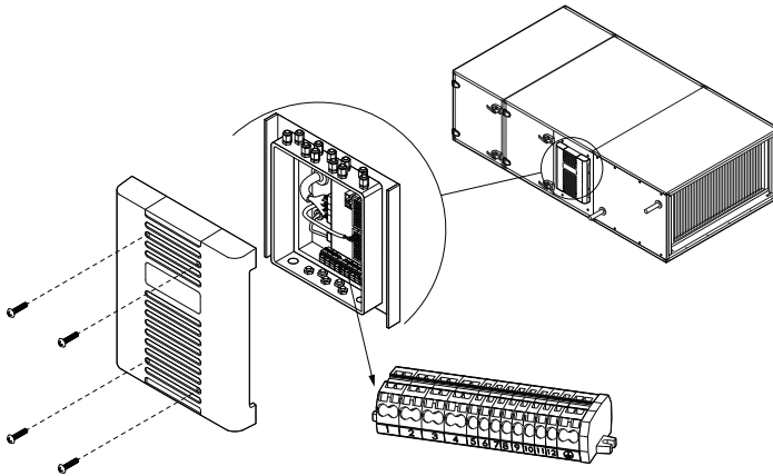
Abb. 47. Anschlussklemmen der Lüftungsgeräte VERSO RA
