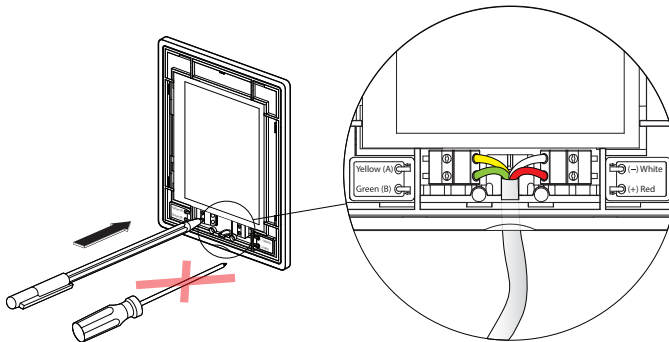
Abb. 50. Anschlussplan für das Bedienpanel
