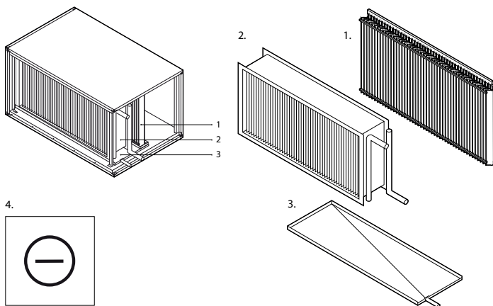
Abb. 6. Abschnitt Kühler
