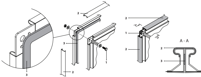
Abb. 32. Beispiel für die Befestigung und Abdichtung eines Flansch-Kanalanschlusses 1 – Schraube, 2 – C-Profil zur Verbindung von Flanschen, 3 – Klebe-Dichtung
