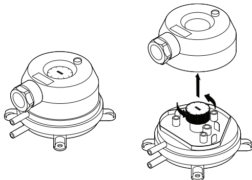
Fig. 2. Der Drucksensor
