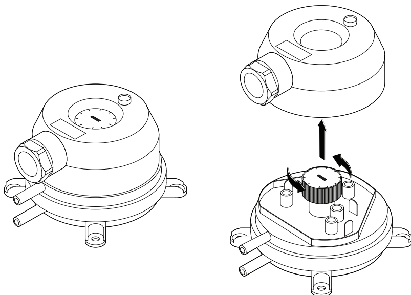
Fig. 2. Der Drucksensor
