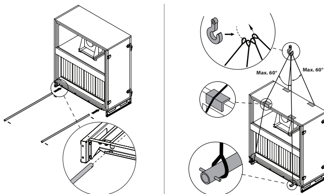
Abb. 14. Anheben einzelner Abschnitte 1
