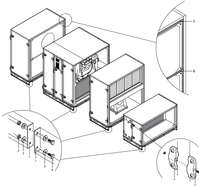
Abb. 21. Äußerer Anschluss und Abdichtung der Abschnitte
