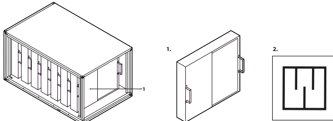
Abb. 10. Abschnitt Lärmunterdrückung
