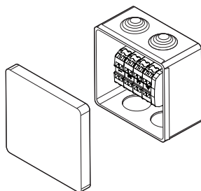
Abb. 49. Verteilerkasten PD1
