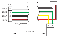
Abb. 46. Anschlussplan für das Bedienpanel
