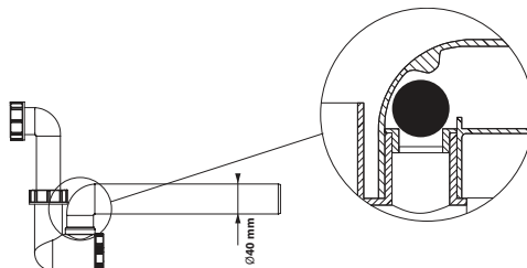
Abb. 29. Beispiel eines Siphons mit Rückschlagventil
