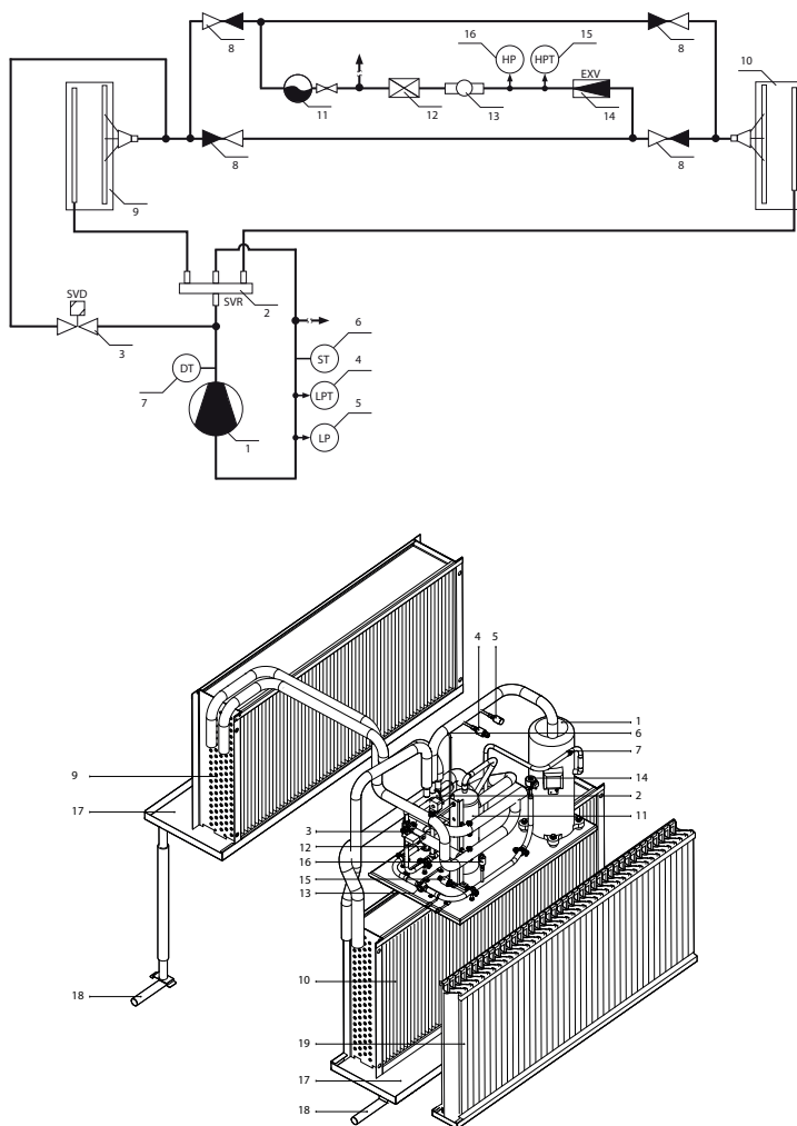
Abb 4. Hydraulischer Schaltplan und Komponenten der Wärmepumpe
