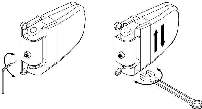
Abb. 20. Einstellen der Scharniere
