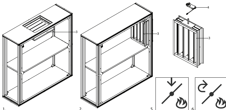
Abb. 12. Abschnitt Rauchabzug
