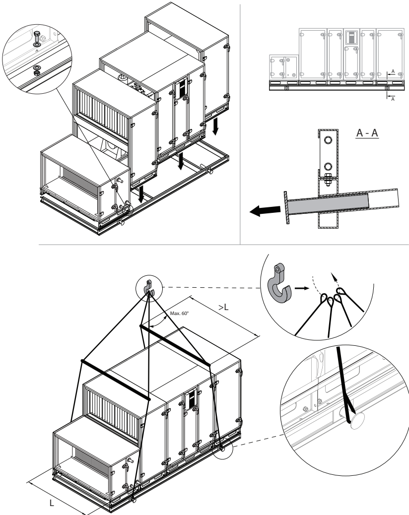
Abb. 15. Vollständig montierte Lüftungsanlage auf verstärkten Sockelrahmen heben 1
