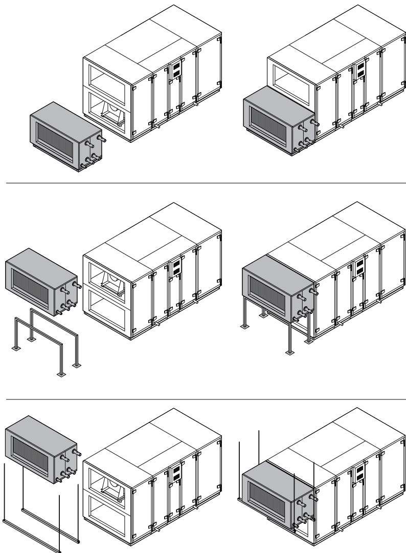
Abb. 24. Beispiele für die Installation von Heiz-/Kühlabschnitten
