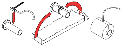
Abb. 26. Installation eines oberflächenmontierten Rücklauf-Wassertemperaturfühlers 2
