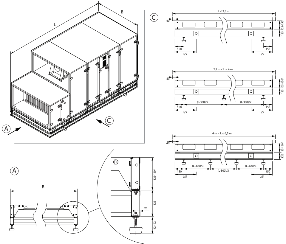
Abb. 16. Abmessungen des verstärkten Montagerahmens
