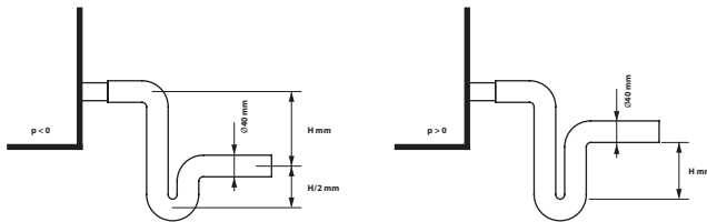
Abb. 28. Installation eines Siphons ohne Rückschlagventil
