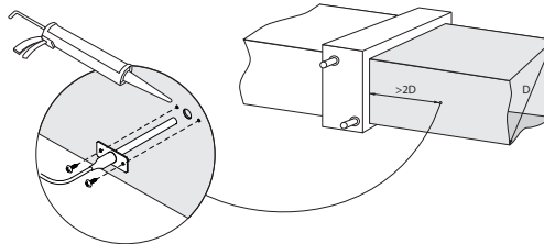
Abb. 43. Installation eines Zulufttemperaturfühlers
