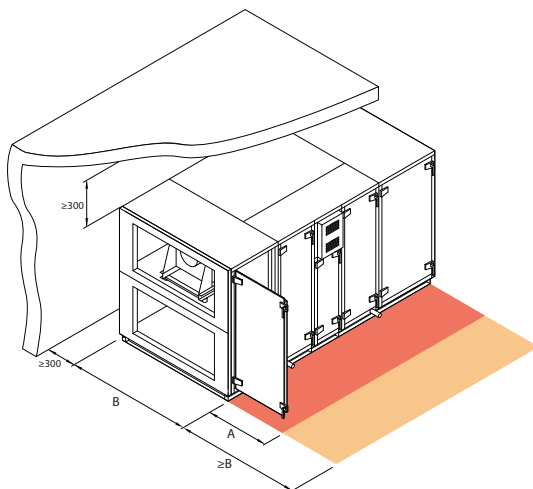
Abb. 18. Inspektionsbereich für Geräte
