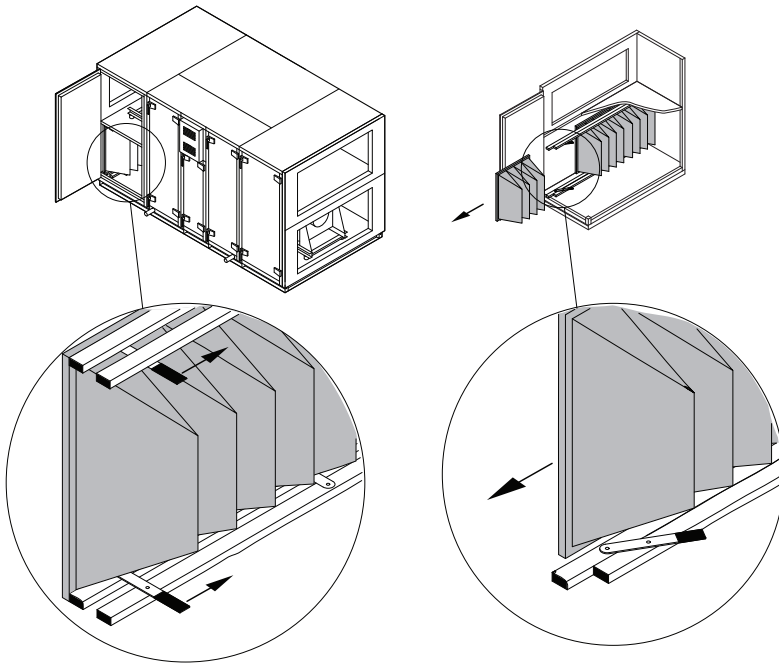
Abb. 53. Filter-Klemmvorrichtung
