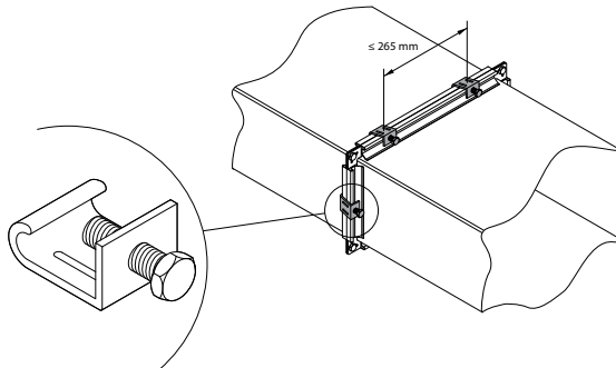
Abb. 32. Beispiel für eine Kanalverbindung mit Kanalklammern
