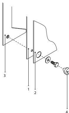
Abb. 23. Interne Verbindung in einem Ventilatorabschnitt
