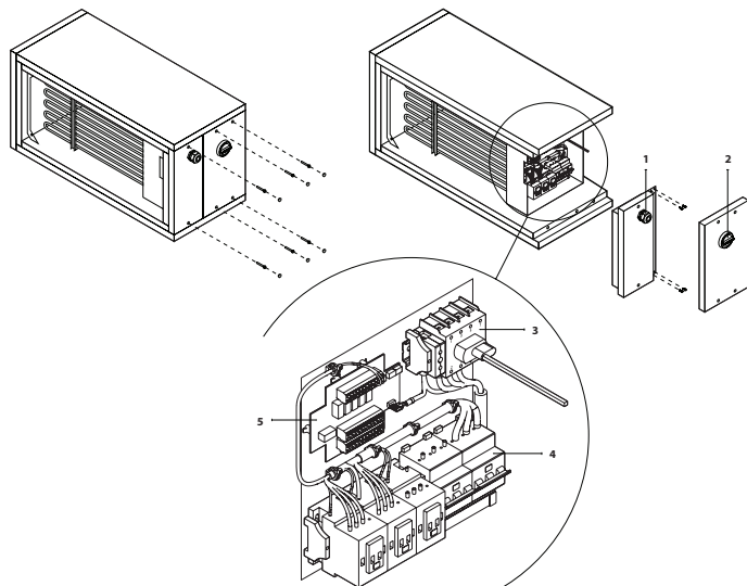
Abb. 36. Haupttrennschalter in elektrischem Heizabschnitt
