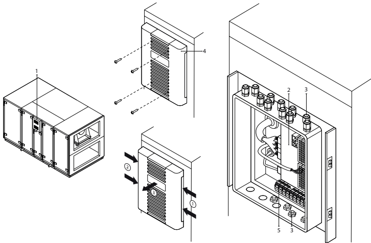
Abb. 37. Steuerungsbox
