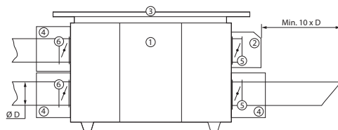
Abb. 33. Zubehör für außen installierte Geräte
