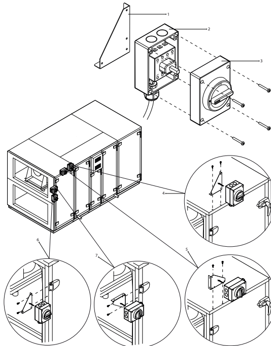
Abb. 35. Hauptleistungsschalter und Montagebeispiele
