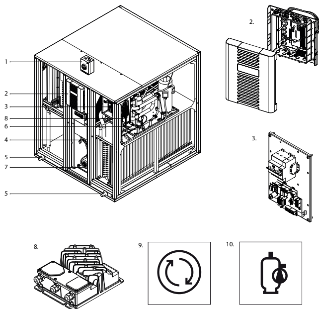
Abb 2. Wärmepumpenbaugruppe
