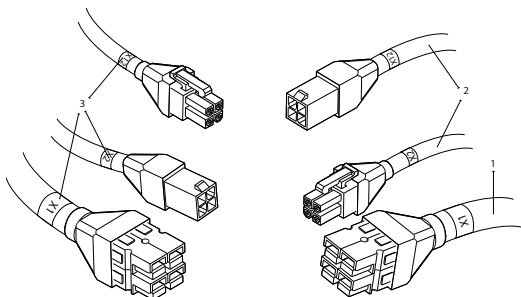
Abb. 48. Kabelverbindungen zwischen Abschnitten
