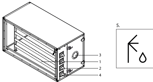
Abb. 11. Abschnitt Luftbefeuchter
