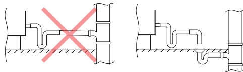
Abb. 30. Anschluss des Kondensatablaufs an die Kanalisation
