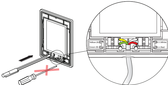
Abb. 47. Anschlussplan für das Bedienpanel
