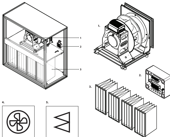
Abb. 1. Filter-Ventilator-Teil
