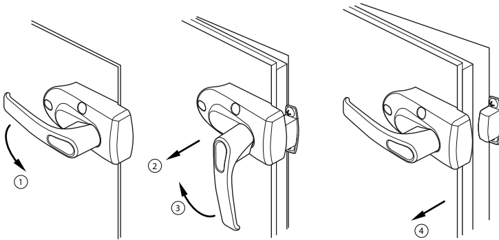
Abb. 19. Öffnen der Tür
