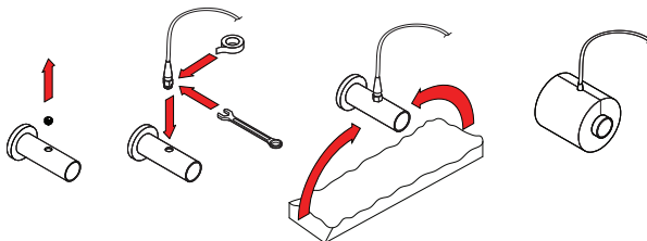
Abb. 27. Installation eines Rücklaufwassertemperaturfühlers mit Gewinde 3
