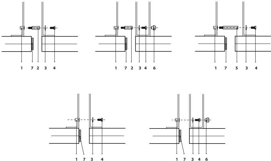
Abb. 22. Arten von internen Abschnittsverbindungen
