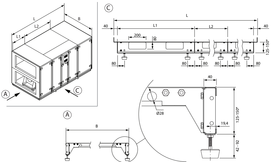
Abb. 17. Einbaurahmen mit verstellbaren Füßen
