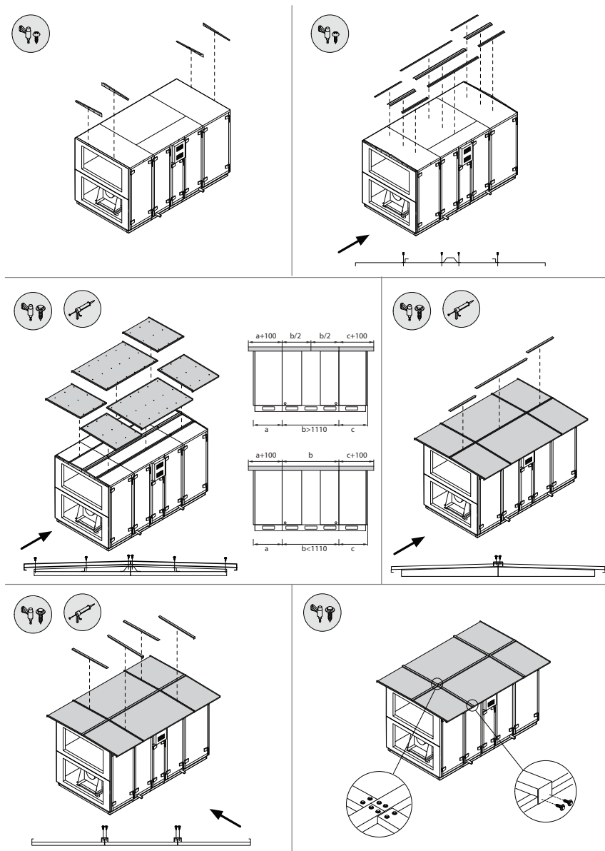
Abb. 34. Installation eines zusätzlich bestellten Schutzdachs 1
