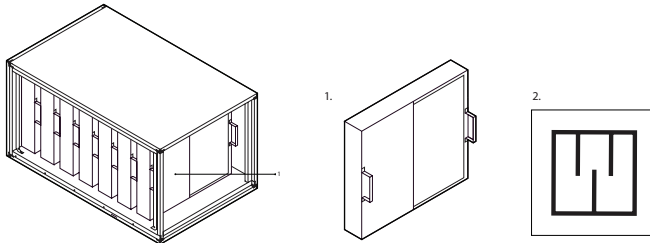
Abb. 10. Abschnitt Lärmunterdrückung
