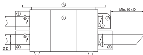
Abb. 28. Zubehör für außen installierte Geräte
