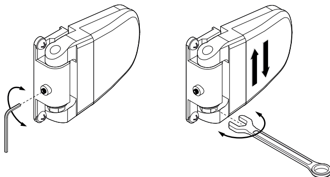
Abb. 16. Einstellen der Scharniere
