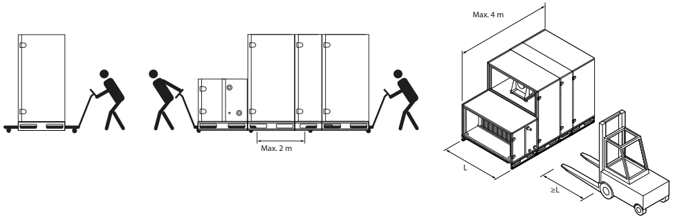
Abb. 11. Transport der Anlage mit einem Gabelstapler oder einem Rollwagen
