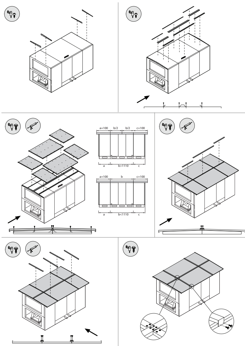
Abb. 29. Installation eines zusätzlich bestellten Schutzdachs 1
