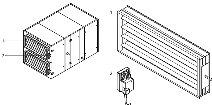
Abb. 9. Luftabsperklappen
