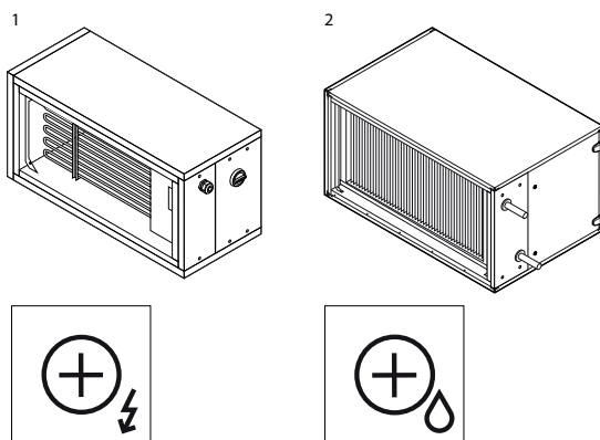
Abb. 8. Abschnitt Erhitzer
