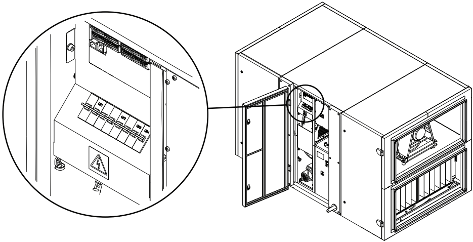
Abb. 32. Standort der Automatisierungsbox
