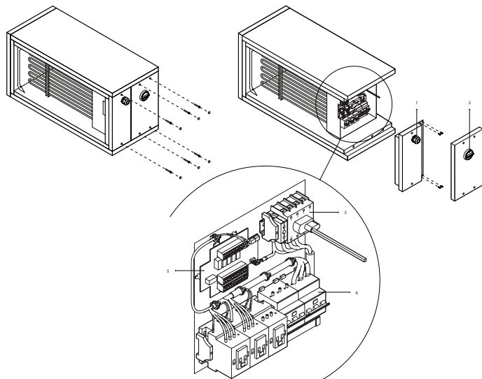
Abb. 31. Haupttrennschalter in elektrischem Heizabschnitt
