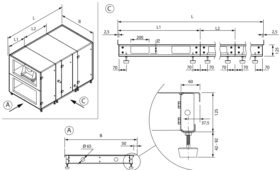
Abb. 15. Einbaurahmen mit verstellbaren Füßen
