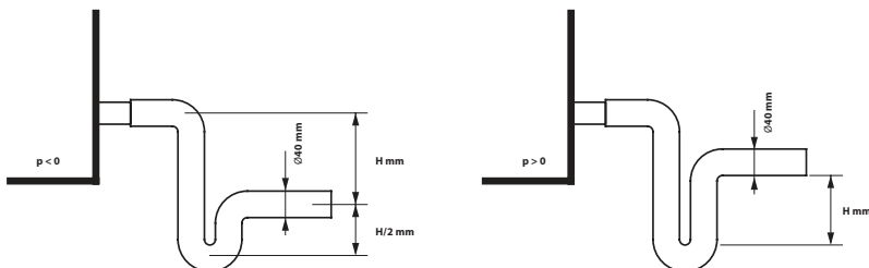
Abb. 23. Installation eines Siphons ohne Rückschlagventil
