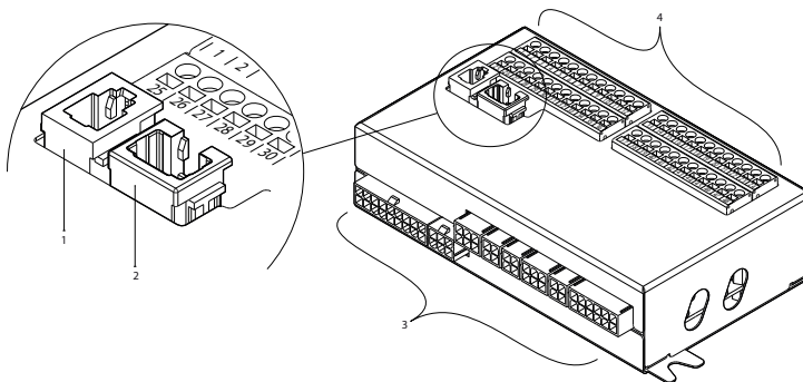
Abb. 33. Hauptplatine des C5-Bedienfeldes
