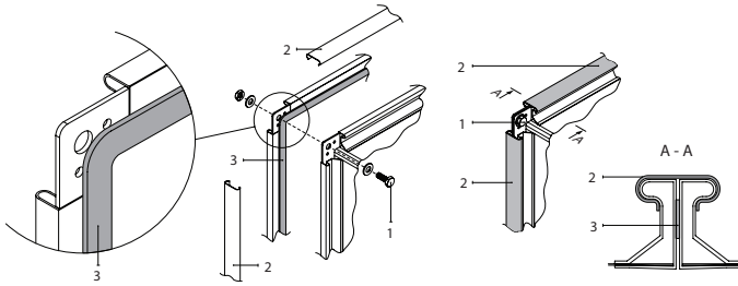
Abb. 26. Beispiel für die Befestigung und Abdichtung eines Flansch-Kanalanschlusses 1 – Schraube, 2 – C-Profil zur Verbindung von Flanschen, 3 – Klebe-Dichtung
