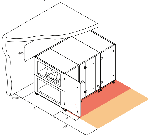
Abb. 17. Inspektionsbereich für Geräte
