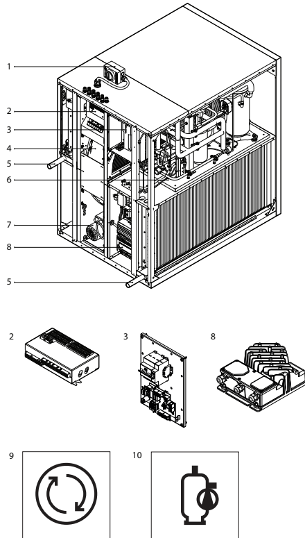
Abb 2. Wärmepumpenbaugruppe
