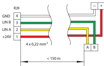
Abb. 39. Anschlussplan für das Bedienpanel
