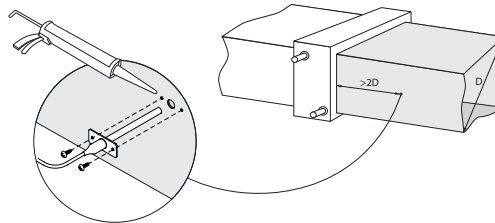
Abb. 38. Installation eines Zulufttemperaturfühlers
