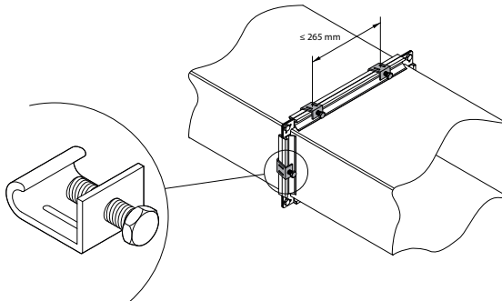
Abb. 27. Beispiel für eine Kanalverbindung mit Kanalklammern
