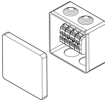
Abb. 42. Verteilerkasten PD1
