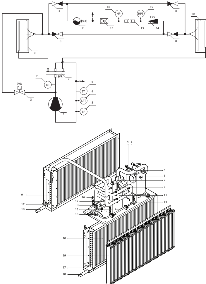
Abb 4. Hydraulischer Schaltplan und Komponenten der Wärmepumpe
