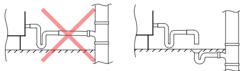
Abb. 25. Anschluss des Kondensatablaufs an die Kanalisation
