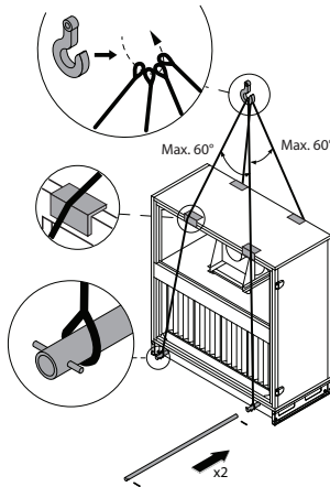
Abb. 12. Anheben einzelner Abschnitte 1
