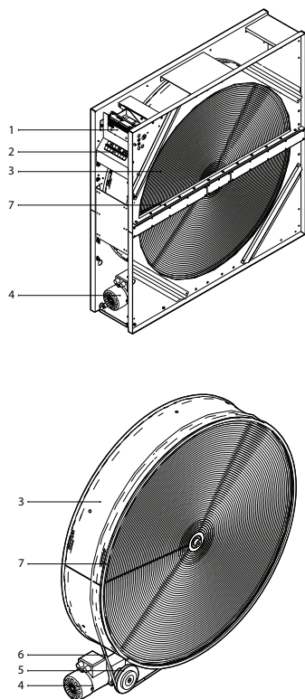
Abb 3. Baugruppe Rotierender Wärmetauscher
