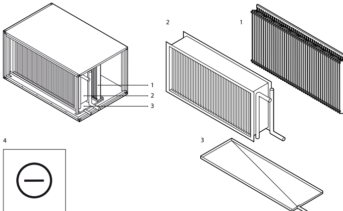
Abb. 7. Abschnitt Kühler 1 – Tropfenabscheider, 2 – Vor-/Rücklauf Register, 3 – Kondensatwanne, 4 – Abschnitt Kühler Kennzeichnung
