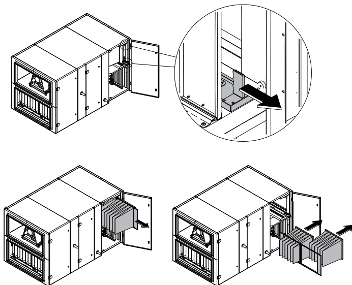
Abb. 46. Filter-Klemmvorrichtung
