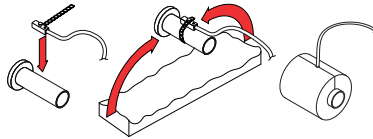
Abb. 21. Installation eines oberflächenmontierten Rücklauf-Wassertemperaturfühlers 2
