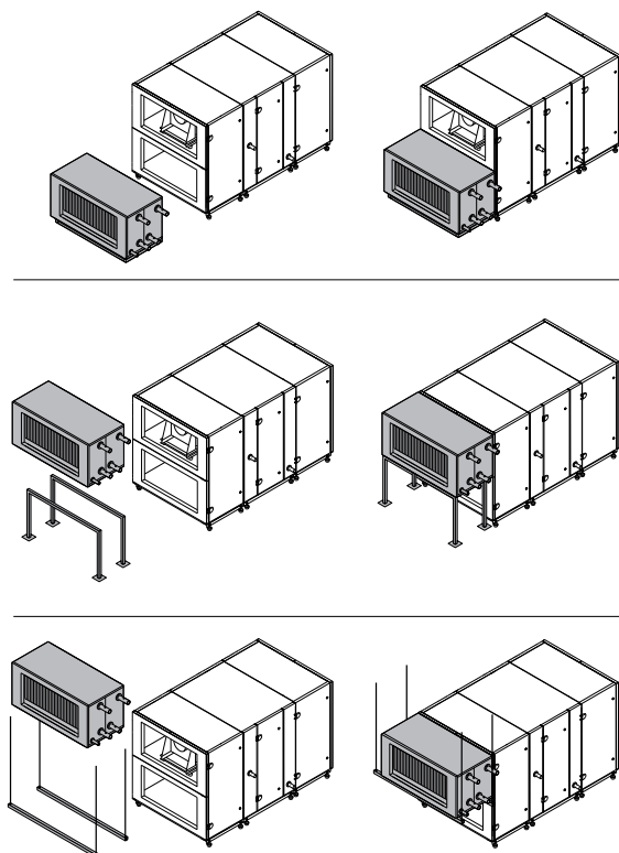
Abb. 19. Beispiele für die Installation von Heiz-/Kühlabschnitten
