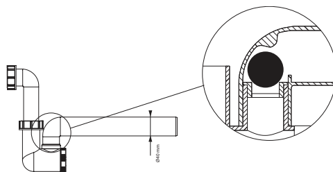
Abb. 24. Beispiel eines Siphons mit Rückschlagventil
