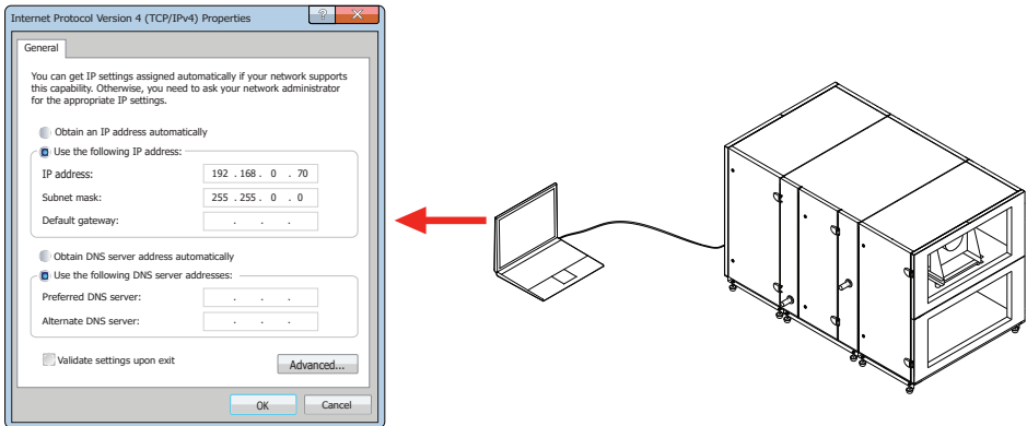
Abb. 44. Computernetzeinstellungen für den direkten Anschluss an das Gerät
