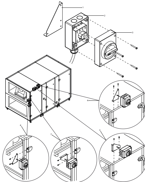
Abb. 30. Hauptleistungsschalter und Montagebeispiele
