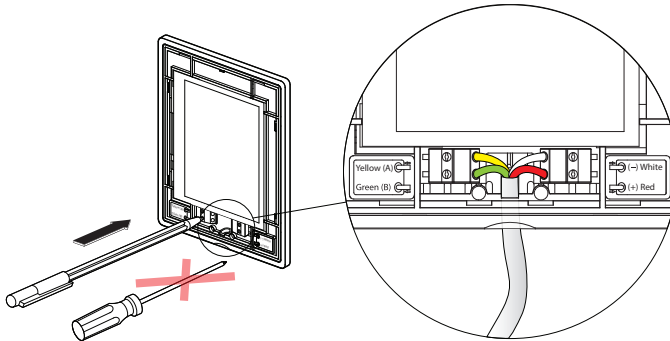
Abb. 40. Anschlussplan für das Bedienpanel
