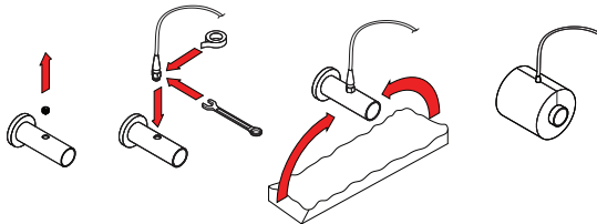
Abb. 22. Installation eines Rücklaufwassertemperaturfühlers mit Gewinde 3
