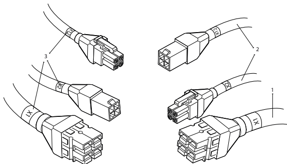
Abb. 41. Kabelverbindungen zwischen Abschnitten
