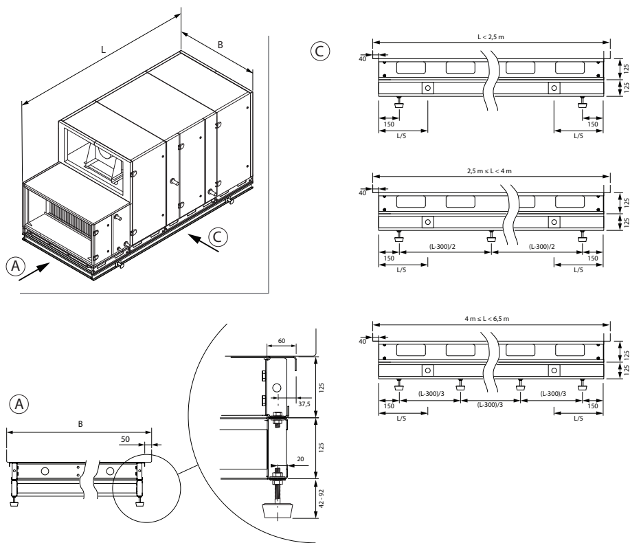
Abb. 14. Abmessungen des verstärkten Montagerahmens
