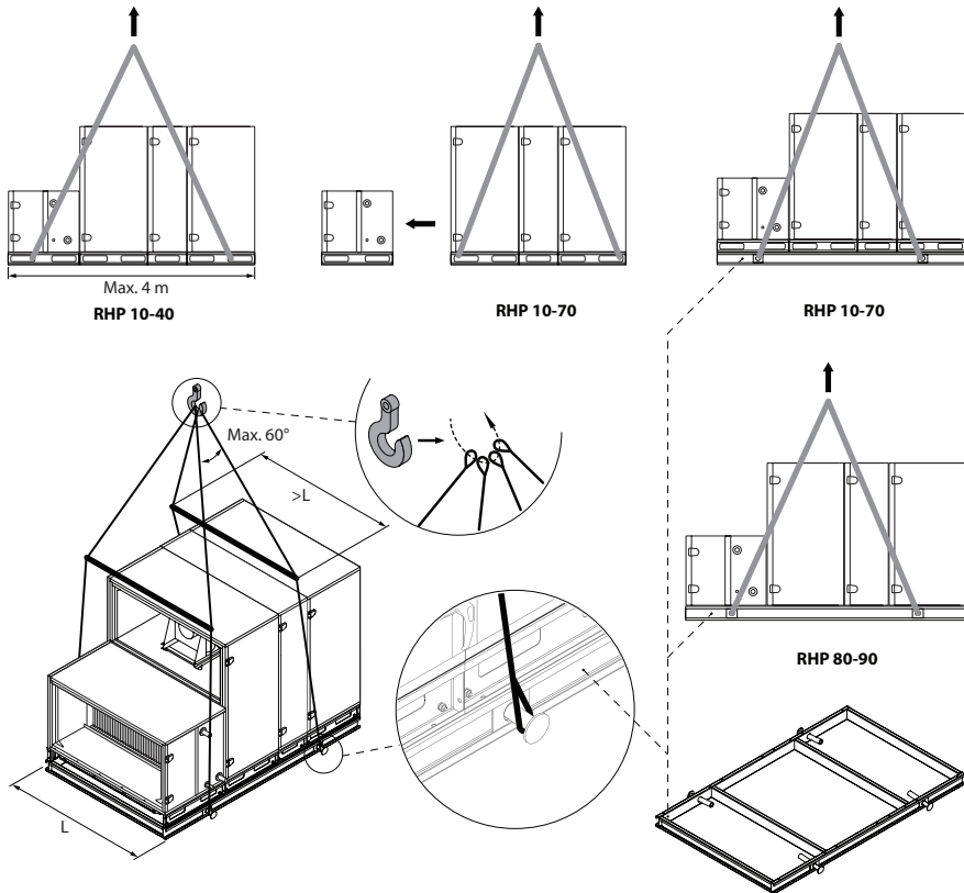
Abb. 13. Anheben der montierten Maschine mit dem Kran 1
