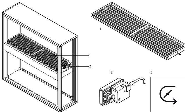
Abb. 6. Abschnitt Umluftsteuerung 1 – Umluftklappe, 2 – Klappenantrieb, 3 – Kennzeichnung der Umluftsteuerung
