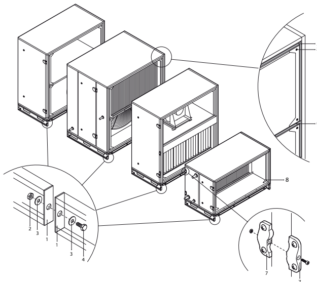
Abb. 18. Äußerer Anschluss und Abdichtung der Abschnitte
