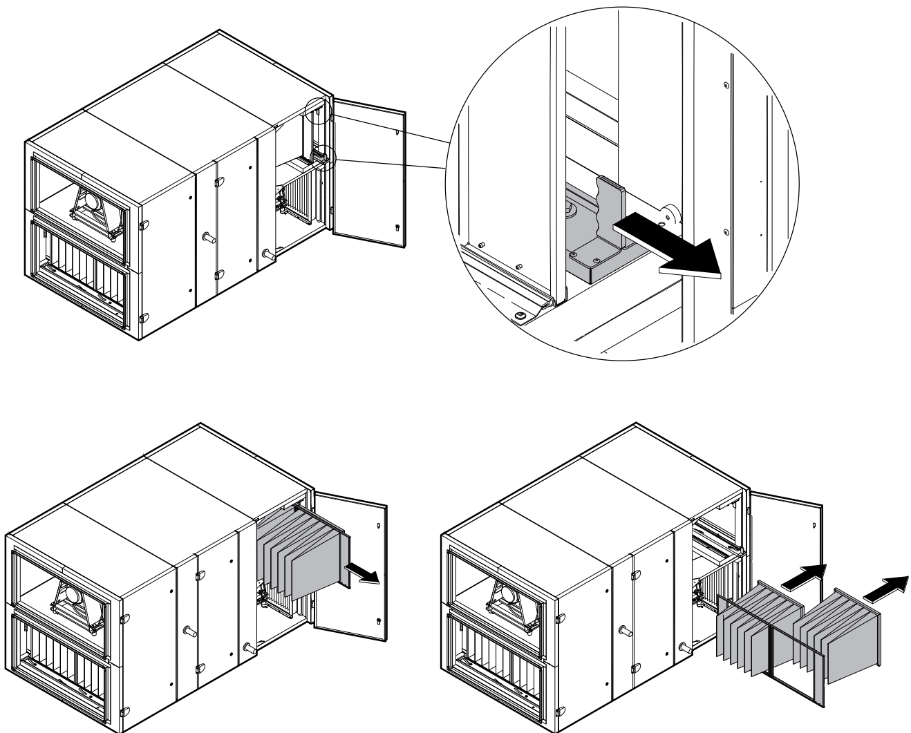
Abb. 3. Filter-Klemmvorrichtung
